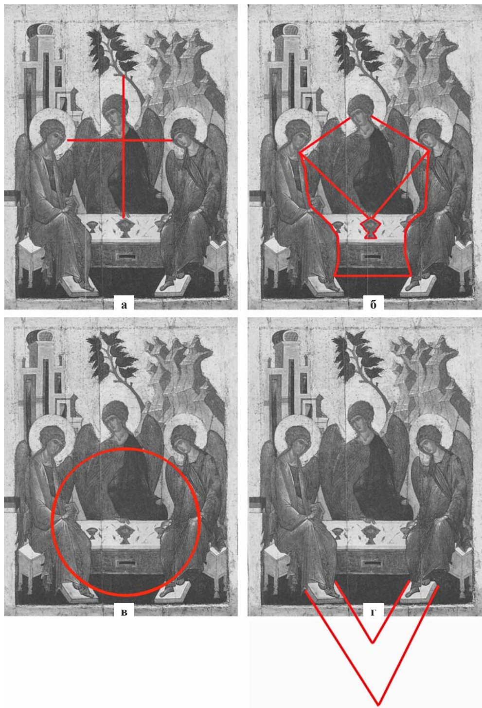
Рис. 5. Пресвятая Троица. Средняя Русь. Середина XVI в. Из Троицкой церкви с. Дивная Гора близ Углича. ЦМиАР: а) образ Этимасии; б) образ чаши; в) композиция вписана в круг; г) линии схода перспективы
